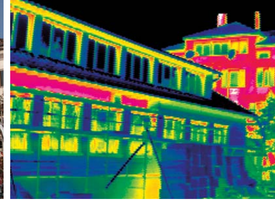
Dämmarbeiten im Gange mit dem bloßen Auge.....und mit dem Infrarotauge der Thermografiekamera
